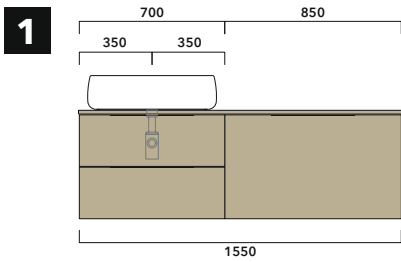
1a | prof./depth cm 37: n.1 BX808 + n.1 BX426 + BXPR38 cm 155
