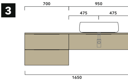
3a | prof./depth cm 37: n.1 BX424 + n. 1 BX994 + BXPR38 cm 165
