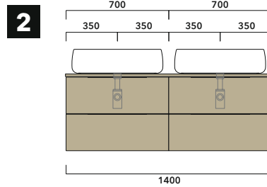
2a | prof./depth cm 37: n.2 BX808 + BXPR38 cm 140
