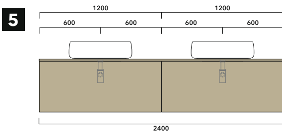
5a | prof./depth cm 37: n.2 BX944 + BXPR38 cm 240
