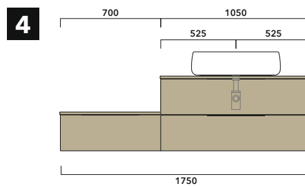
4a | prof./depth cm 37: n.1 BX296 + n. 1 BX838 + BXPR38 cm 70 + BXPR38 cm 105
