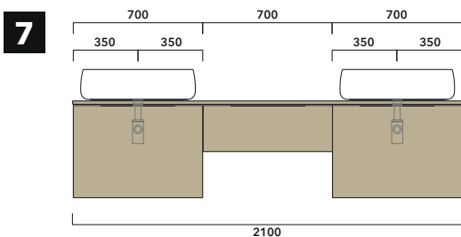
7a | prof./depth cm 37: n.2 BX804 + n. 1 BX296 + BXPR38 cm 210
