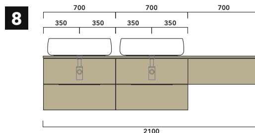
8a | prof./depth cm 37: n.2 BX808 + n. 1 BX296 + BXPR38 cm 210
